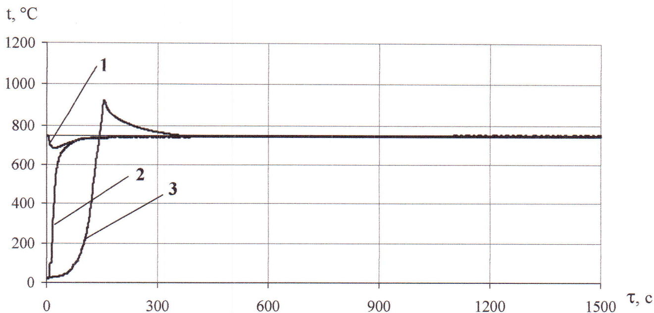
Рисунок 1 - Характерний графік змінення температури у печі (1), на поверхні (2) та всередині (3), зразків мінераловатної теплоізоляційної плити марки «ТЕХНОРУФ ПРОФ», виробництва ТОВ "Завод теплоізоляційних матеріалів "ТЕХНО", під час випробувань згідно з ДСТУ Б В.2.7-19-95 (ГОСТ 30244-94).
