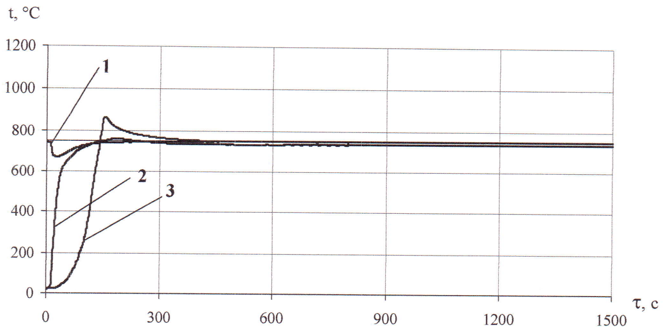
Рисунок 1 - Характерний графік змінення температури у печі (1), на поверхні (2) та всередині (3), зразків мінераловатної теплоізоляційної плити марки «ТЕХНОРУФ В ОПТИМА» виробництва ТОВ "Завод теплоізоляційних матеріалів "ТЕХНО", під час випробувань згідно з ДСТУ Б В.2.7-19-95 (ГОСТ 30244-94).
