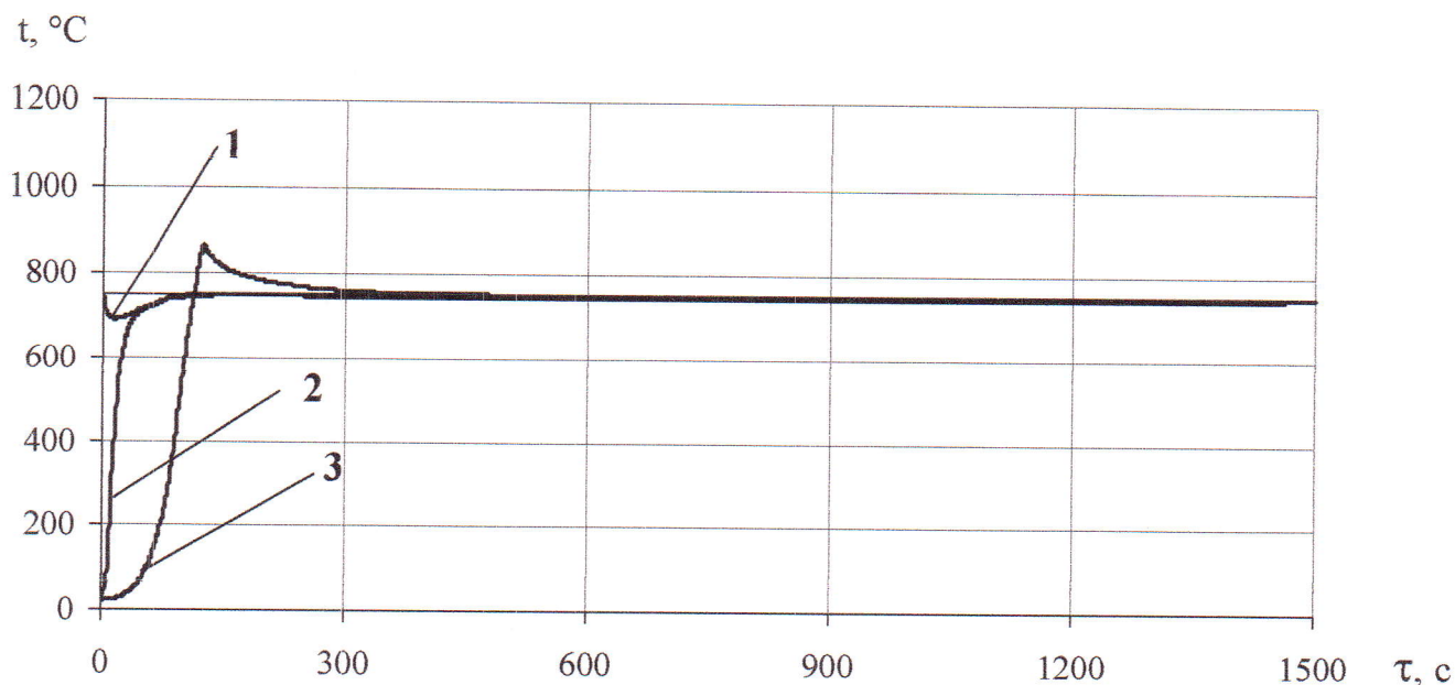
Рисунок 1 - Характерний графік змінення температури у печі (1), на поверхні (2) та всередині (3), зразків мінераловатної теплоізоляційної плити марки «ТЕХНОФАС ОПТИМА» виробництва ТОВ "Завод теплоізоляційних матеріалів "ТЕХНО", під час випробувань згідно з ДСТУ Б В.2.7-19-95 (ГОСТ 30244-94).
